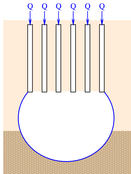
Groupement de pieux la zone compressible est influencée par l'effet radier du groupe de pieux
